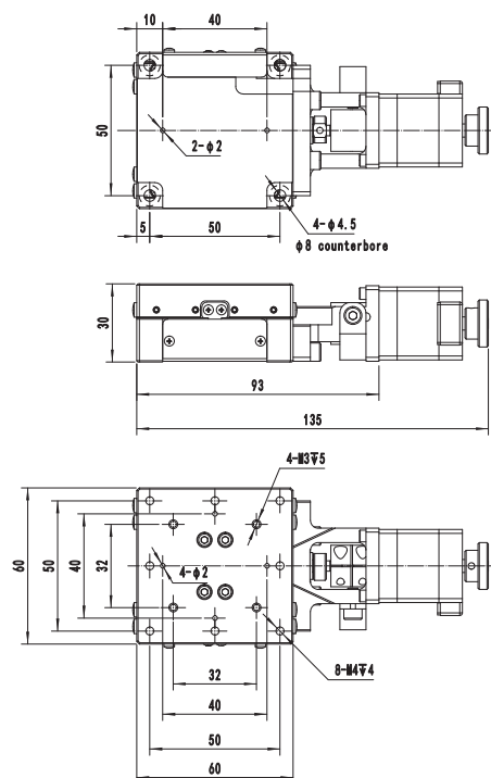
CXPF50-80100
